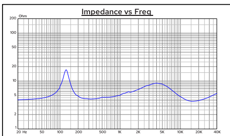
阻抗曲线
