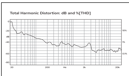
失真曲线
